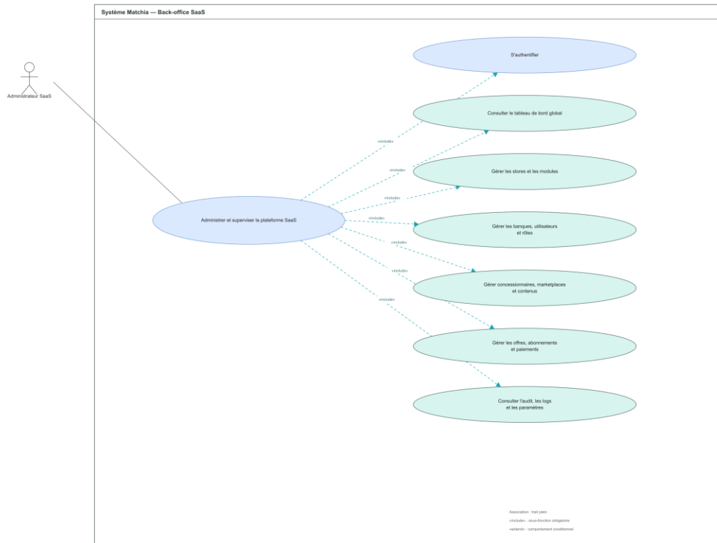
Figure 3.4 — Diagramme de cas d'utilisation détaillé : Administrer et superviser la plateforme SaaS
